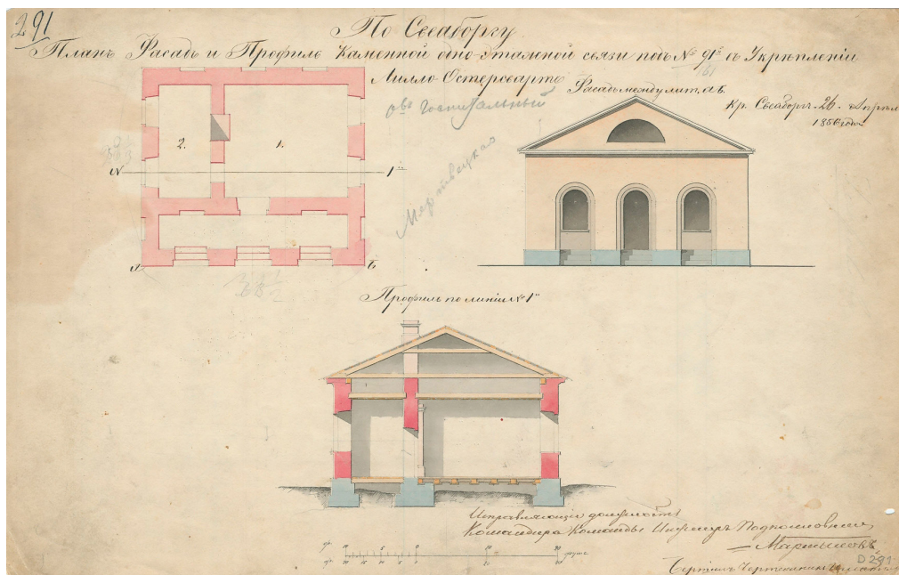
Ruumishuoneen suunnitelupiirustukset vuodelta 1856.
